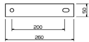
連結用プレート 6X50X260
